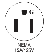
NEMA 5-15P
